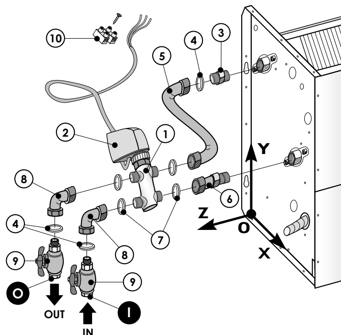
POSIZIONE ATTACCHI IDRAULICI (AD INSTALLAZIONE ULTIMATA) WATER CONNECTIONS POSITION (WHEN THE INSTALLATION IS FINISHED)
