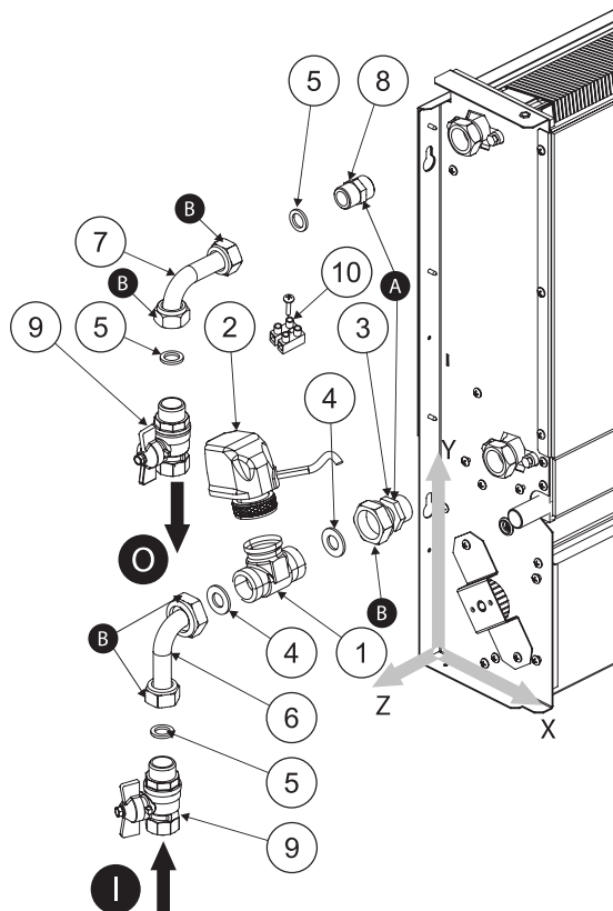
Posizione attacchi idraulici (ad installazione ultimata) Water connections position (when the installation is finished)
