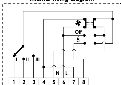
Schema elettrico interno Internal wiring diagram
